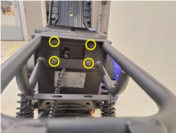
Löysää takapenkin rungon kiinnityspultit (kiintoavain 12 mm).
